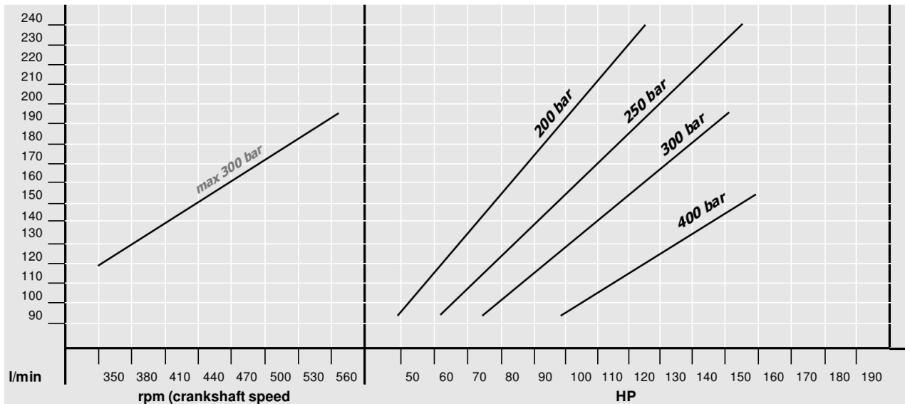
Grafico potenza/pressioni. Performance curve. Diagramme puissance/pressions
